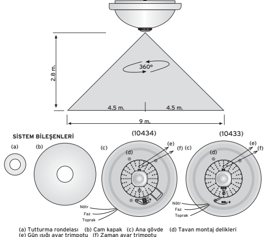
(a) Tutturma rondelası (b) Cam kapak (c) Ana gövde (d) Tavan montaj delikleri (e) Gün ışığı ayar trimpotu (f) Zaman ayar trimpotu
